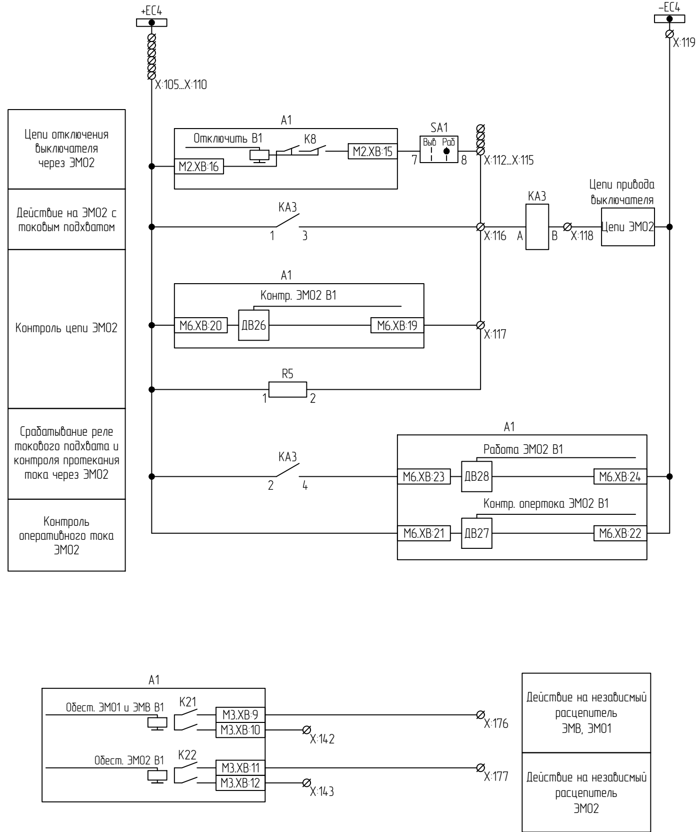
Цепи ЭМ02
